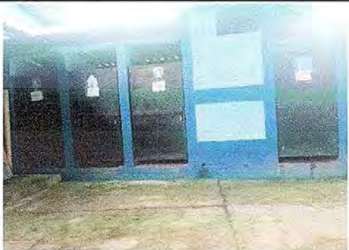
Foto No. 21, Módulo No. 4. Mantenimiento a estructura de puerta (lijado, cambio de tubo. Cepillado, sujeción, aplicación de pintura
