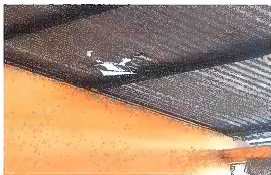
Foto 5: MODULO 4 SUSTITUCION DE LAMINA POR LAMINA TROQUELADA ALUZINC CALIBRE 26
