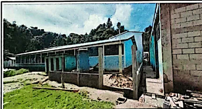
Foto 5: Reparación de muro perimetral con block y tubo HG
