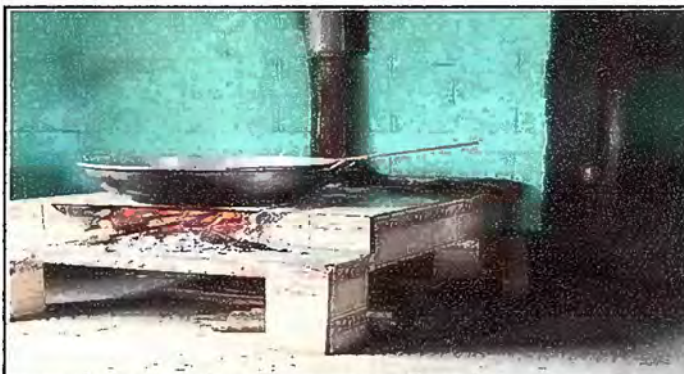
Foto 4. Módulo 2 sustitución de chimenea de concreto
