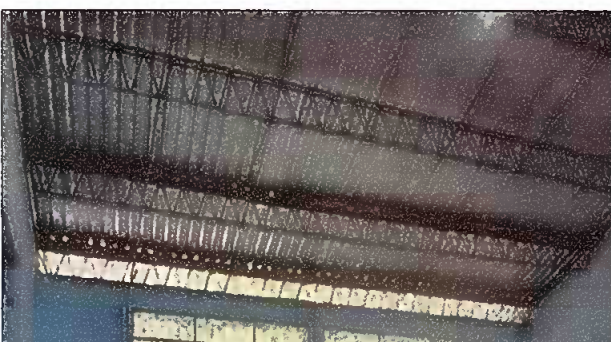
Foto 6: MODULO 1. Sustitucion de laminas, por lamina troquelada aluzinc calibre 26
