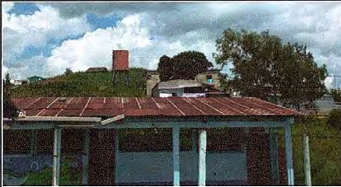
Foto 1: MODULO 1. Sustitución de lámina por lámina troquelada. Sustitución de canal.
