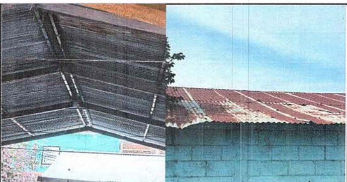
Foto 13: MODULO 3 Sustitución de lámina por lámina troquelada Aluzinc calibre 26, Sustitución de capote de lámina por lámina troquelada, sustitución de elementos de fijación (tornillos) desinstalación de lámina
