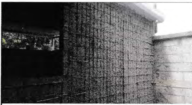
Foto 4: Colocación de muro perimetral en Aula
