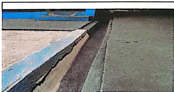
foto 4 reparación de cuneta
