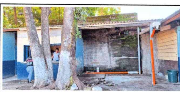
Foto 6: Instalacion de Estructura Metalica para nueva Galera para ampliacion de cocina.
