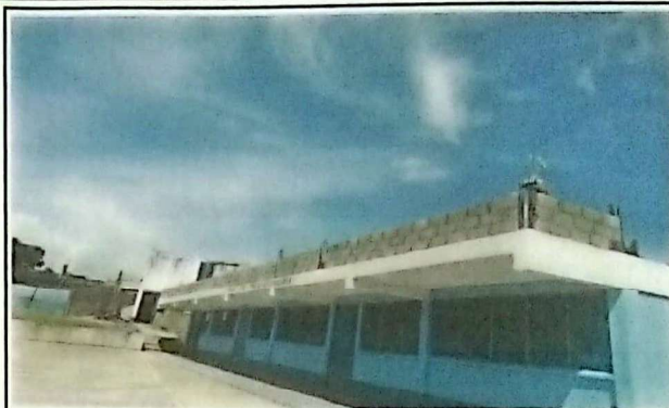
Foto 2: Suministro de estructura metálica de cancha Construcción de pared para soporte de la estructura metálica
