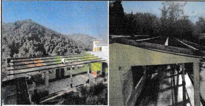
Foto 1: RETIRO DE LÁMINAS ANTIGUAS MODULO 1 Y MODULO 2
