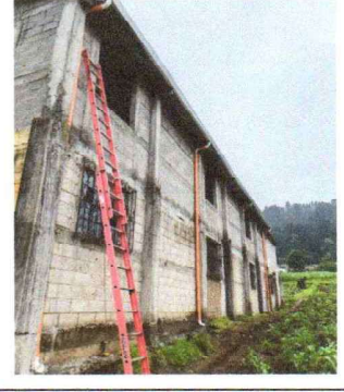
Foto 2: VISTA DE INSTALACIÓN DE CANALES Y BAJADA DE AGUA PLUVIAL, FINALIZADO
