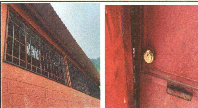
Foto 4: VISTA DE INSTALACIÓN DE BALCON Y SUSTITUCIÓN DE CHAPA YALE FINALIZADO
