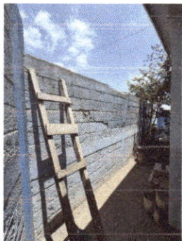
Foto 7: MURO PERIMETRAL DAÑADO, PRESENTA FISURAS Y ESTA CON DESPLOME
