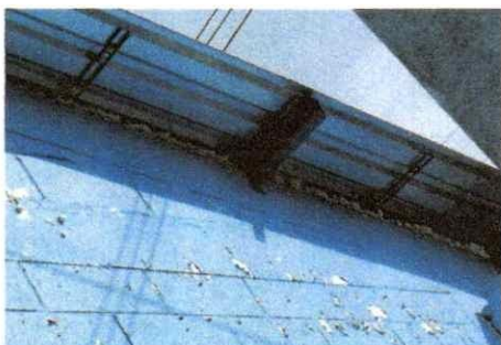
Foto1: Suministro e instalación de costaneras galvanizadas de 2x4 y tubo rectangular de 1x2 para darle resistencia a las láminas y sellar para evitar ingreso de aves
