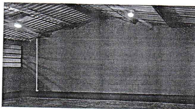
Foto 4: Finalizacion de la colocacion de la estrucuta portante de metal para refuerzo de techo modulo no.2
