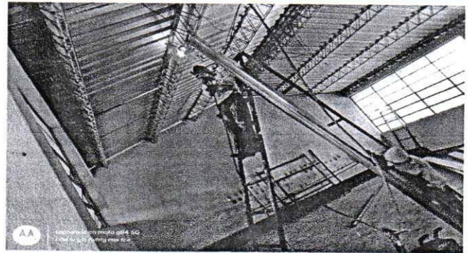
Foto 4: Colocacion de estructura portante de metal para refuerzo de techo modulo no.2
