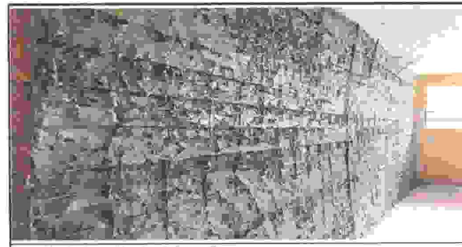
Foto 6: Colocación de electromalla
