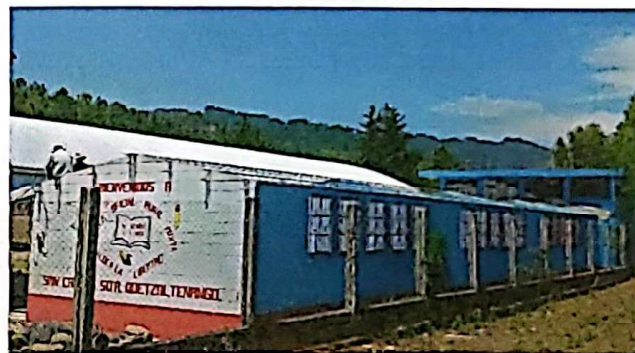
sustitución de lámina, por lamina troquelada calibre 26
