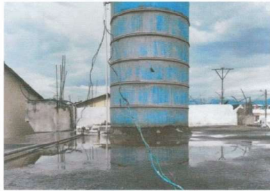
Foto 3: VISTA FINALIZADO CAMBIO ACCESORIOS DEPOSITO DE AGUA FINALIZADO
