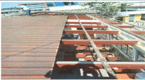
Foto1: RETIRO DE LÁMINAS ANTIGUAS
