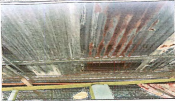
Sustitución de lámina por lámina troquelada aluzinc
