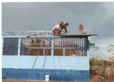
Foto1: Sustitución de lamina, por lamina troquelada aluzinc calibre 26 modulo de aulas
