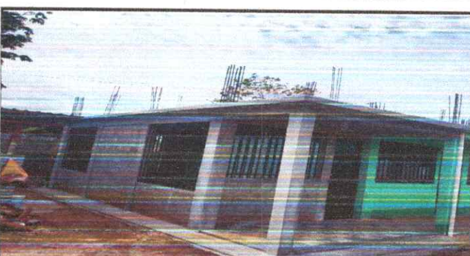
Foto 4: Realización de techo de terraza
