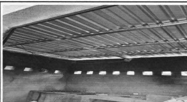
Foto 10: Instalación de lámina troquelada aluzinc calibre 26
