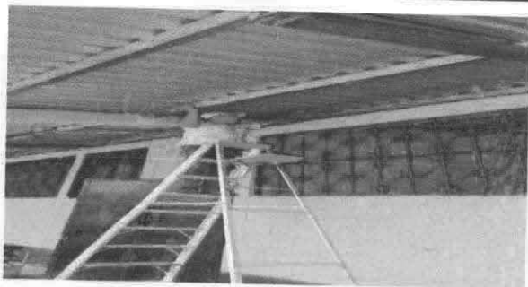
Foto 10: Sustitución de elementos de fijación en cubierta de lámina
