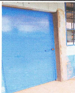
Foto 1: Mantenimiento a estructura (lijado, cambio de tubo, cepillado, sujeciones, aplicación de pintura)
