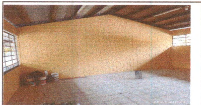
Foto 3: Sustitución de piso liso a piso de granito en las aulas
