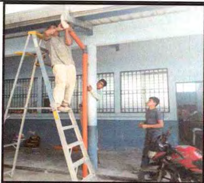
Foto7: Instalación de bajadas de agua pluvial tubo PVC3" en corredor
