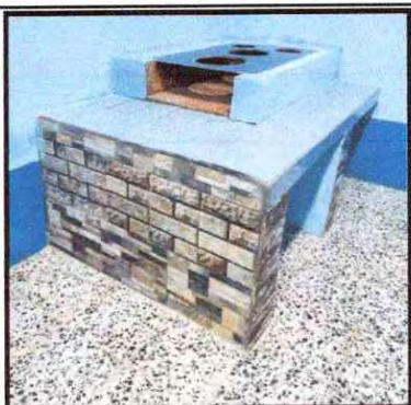
Foto 27: Sustrucción de azulejo en estufa rural completa (plancha y chimenea)
