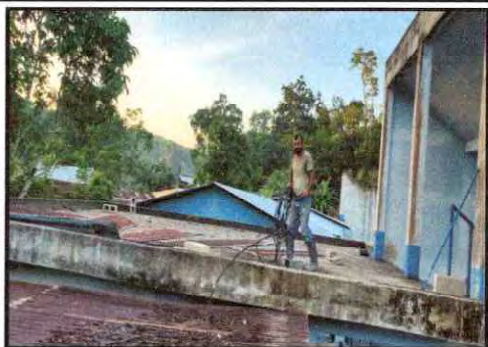
Foto 11: Reparación de cableado eléctrico
