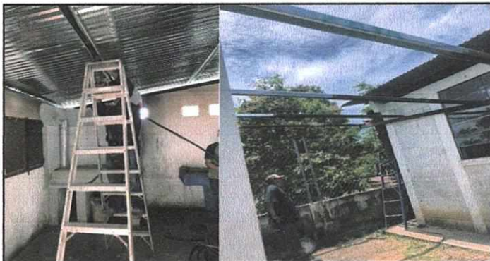
Foto 6: SUSTITUCION DE LAMINA POR LAMINA y MEJORAMIENTO DE ESTRUCTURA DE SOPORTE DE METAL
