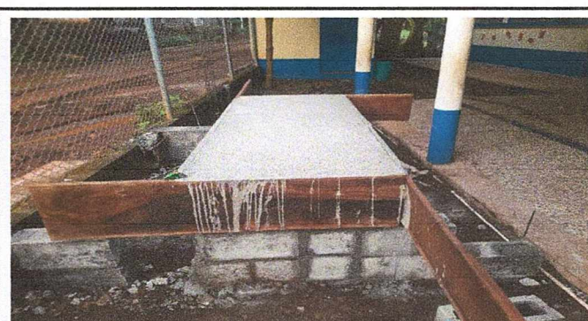
Foto 6: FUNDICION DE SEGUNDA MESA DE CONCRETO.
