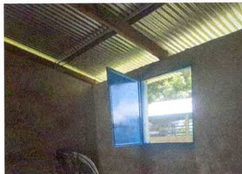
Foto 8: Detalles finales de mantenimiento de ventanas metálica de Aula (lijado, pintura y soldadura)
