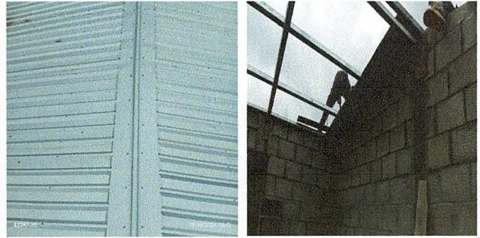
Foto 2: Sustitución de lámina dañada con lámina troquelada calibre 26 y sustitución de estructura dañada con estructura portante galvanizada en techo de cocina.
