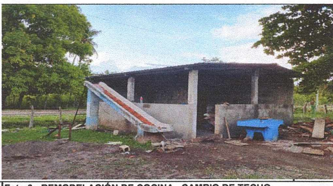
Foto 6: REMODELACIÓN DE COCINA, CAMBIO DE TECHO, ESTRUCTURA Y REPELLO.
