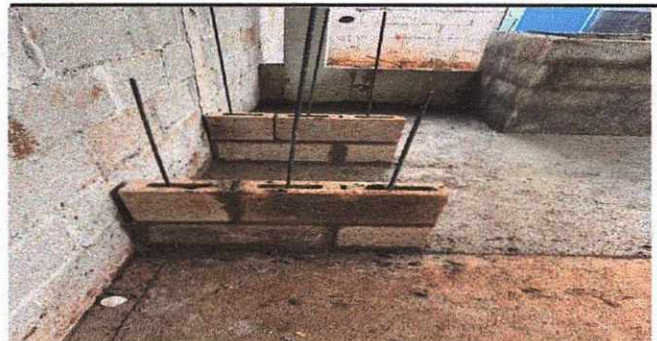
Foto 6: ESTUFA RURAL SUSTITUCION DE ORNILLA A ESTUFA RURAL ELABORADA CON CEMENTO, HIERRO Y BLOCK, PLANCHA DE 4 ORNILLAS, LADRILLO, CAL.
