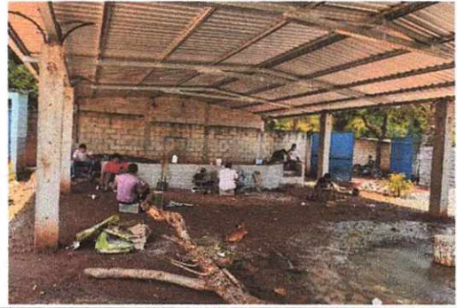
Foto 2: GALERA CON SU RESPECTIVO ESCENARIO, SUSTITUCION DE ESTRUCTURA METALICA, SUSTITUCIÓN DE TECHO, SUSTITUCION DE ESTRUCTURA METALICA, ELABORACION DE ESCENARIO BLOCK,
