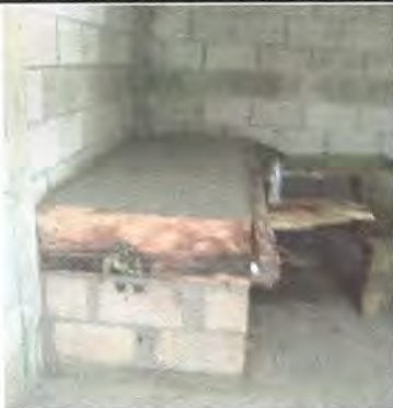
Foto 9: Polleton de block con su respectiva plancha en fase de reforzamiento estructural.
