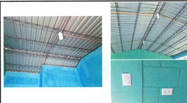
INSTALACIÓN ELÉCTRICA, REPARACION DEL SISTEMA ELÉCTRICO (CABLEADO, TOMAS, APAGADORES Y LUMINARIAS)
