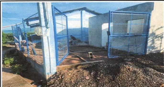
Foto 1: Trabajos de pavimentación en patio, repello en cocina y preparación para colocación de puertas y ventanas.
