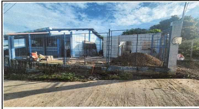
Foto 4: Preparación y trabajos de nivelación para la colocación de techo en área de cocina, baños y patio.
