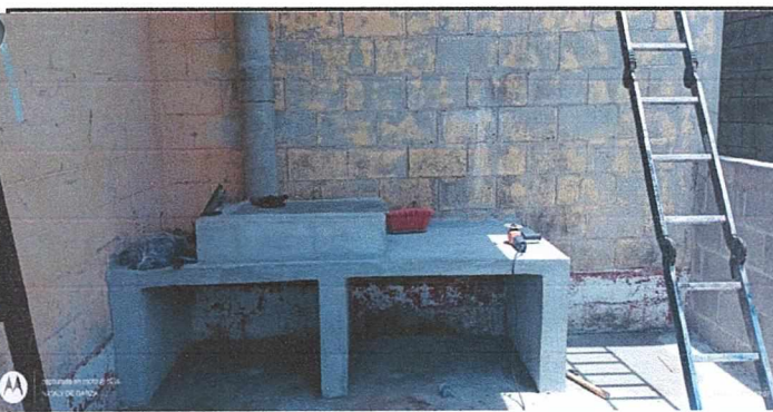
FOTO 5: CONSTRUCCIÓN DE CICINA DE LENA
