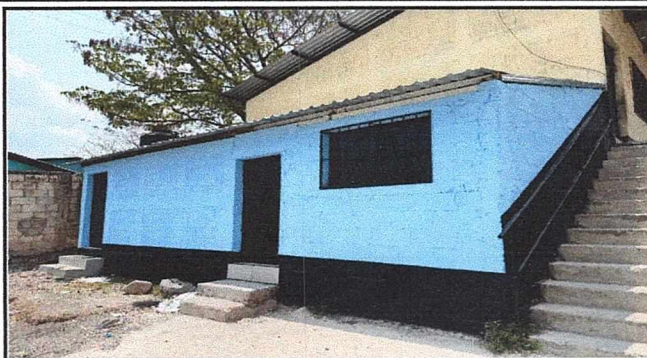
Foto 2: Pintura en muros exteriores, instalación de puerta metálica con chapa y ventana metálica con balcón.
