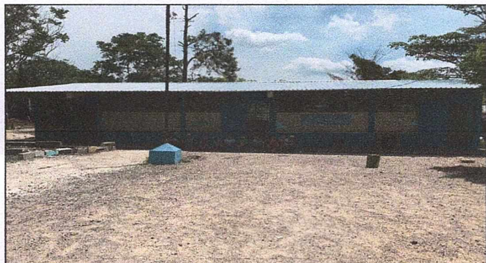
Foto 3: Sustitución de duralita por lamina aluzinc calibre 24
