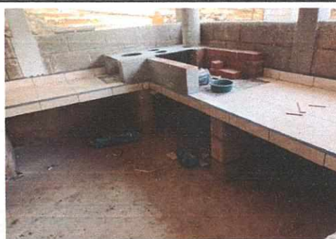
Foto 6: Mesones de cocina, azulejeados ya con las planchas y las chimeneas instaladas.
