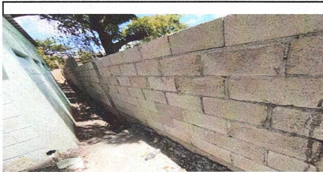
Foto 1: muro de mampostería
