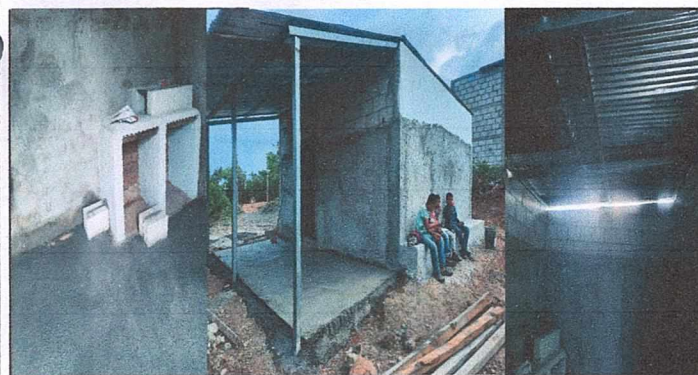
Foto 5: cocina rustica, paredes de adobe, techo con constaneras de madera y torta rustica, se colocará block con sus columnas, techo de estructura galvanizada, repello y torta adentro de la cocina.
