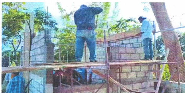
Foto1: Mejoramiento en pared de block
