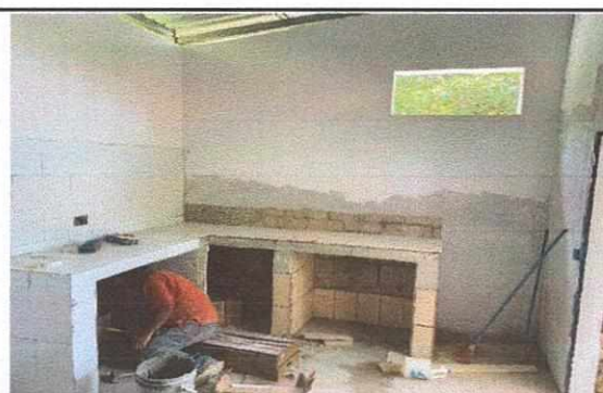
Foto 12: Cernido de paredes e instalación de azulejo y piso cerámico en cocina.
