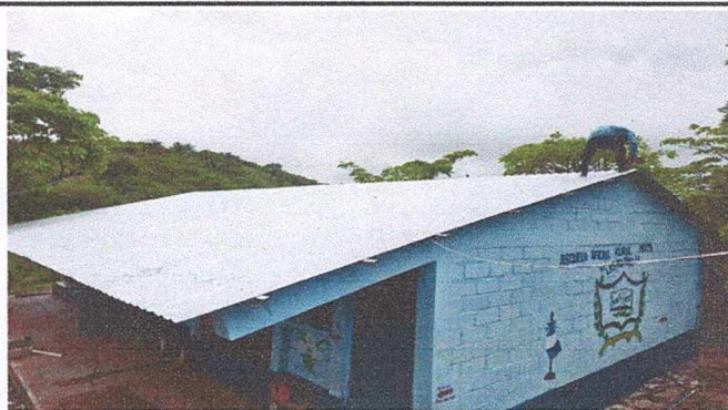
Foto 2: SUSTITUCIÓN TECHO CON DURALITA Y ESTRUCTURA DE METAL POR LÁMINA TROQUELADA EN MODULO DE AULAS
