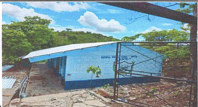
Foto1: SUSTITUCIÓN TECHO CON DURALITA Y ESTRUCTURA DE METAL POR LÁMINA TROQUELADA EN MODULO DE AULAS
